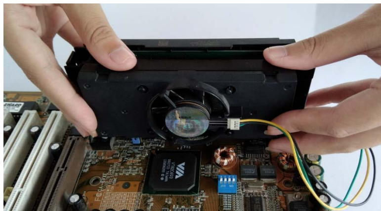
ภาพที่ 5.10 การติดตั้งซีพียูเป็นแบบคาร์ทริดจ์ (Cartridge)
