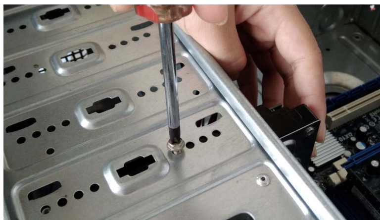
ภาพที่ 5.17 การติดตั้งฮาร์ดดิสก์ลงในเคส
