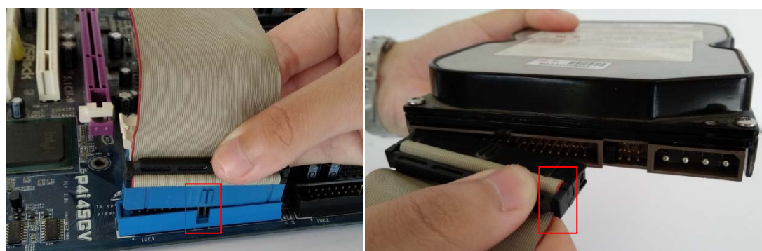
ภาพที่ 5.19 การติดตั้งสายแพบนเมนบอร์ด และฮาร์ดดิสก์
