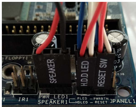
ภาพที่ 5.35 แสดงการเชื่อมต่อสวิทช์ ไฟแสดงผล และลำโพงแจ้งสถานะ บนเมนบอร์ด
