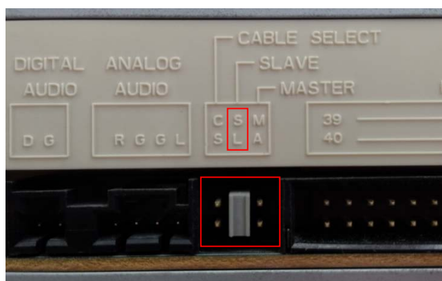
ภาพที่ 5.21 การกำหนดให้อุปกรณ์ออปติคอลไดรฟ์แบบไอดีอีเป็นอุปกรณ์รอง (Slave)
