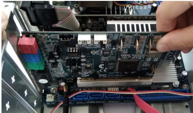
ภาพที่ 5.26 การติดตั้งการ์ดเสียง
