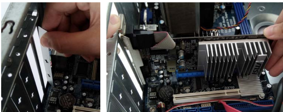
ภาพที่ 5.25 การติดตั้งการ์ดแสดงผล
