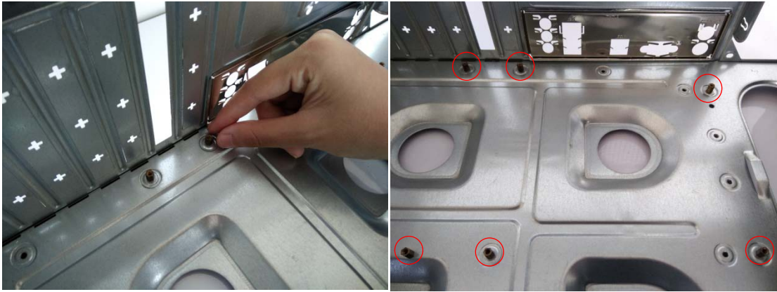
ภาพที่ 5.7 การติดตั้งเสารองเมนบอร์ดบนแท่นรองเมนบอร์ด
