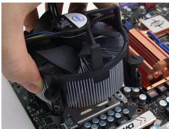
ภาพที่ 14.4 การติดตั้งซีพียูและพัดลมซีพียู
