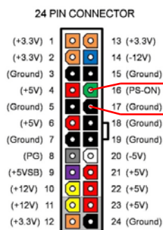
ภาพที่ 14.3 ตำแหน่งการลัดวงจร (Short) หัวต่อแบบเอทีเอ็กซ์ (ATX)
