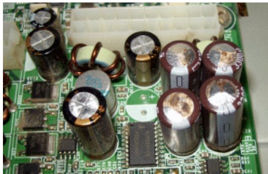
ภาพที่ 14.5 ตัวเก็บประจุบนเมนบอร์ดที่มีลักษณะปูดบวม
