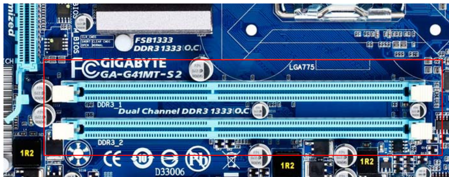
ภาพที่ 11.3 สล็อตแรมบนเมนบอร์ดที่รองรับแรมดีดิดอาร์ 3 (DDR3) บัส 1333 MHz
