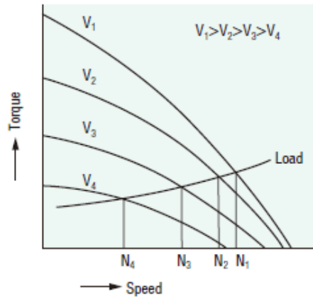
กราฟความสัมพันธ์ระหว่างความเร็ว กับแรงบิดของ มอเตอร์ เมื่อมีโหลด
